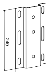
VIKTFÖRDELNINGSPLATTA
