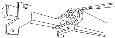
FÖRLÄNGT BÄRRÖR
